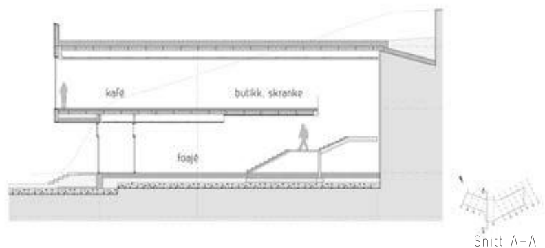
Eksponert fjell i samvirke med plasstøpt betong
