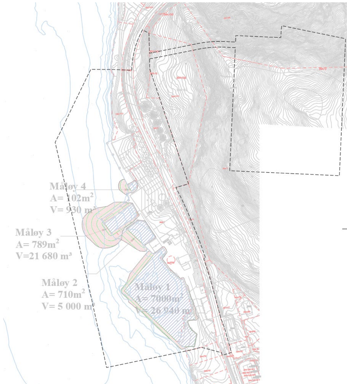
Figur 3 Plangrense med fyllinger
